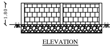
ELEVATION
