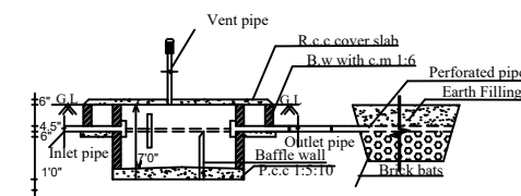
SECTION OF S.P.T & D.T
