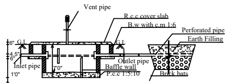
SECTION OF S.P.T & D.T
