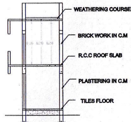
SECTION 'ab'
