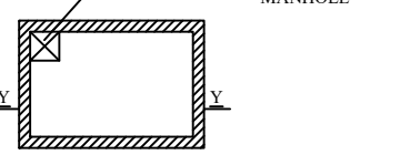
UG - SUMP DATAIL PLAN
