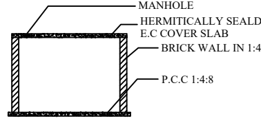
SECTION ON Y - Y
