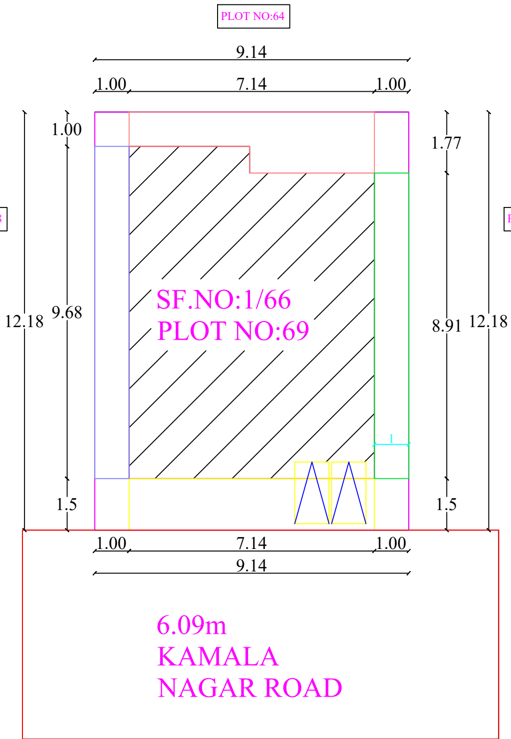
SITE PLAN 1:100
