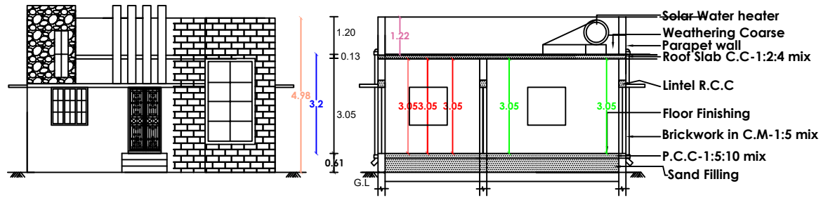
ELEVATION
