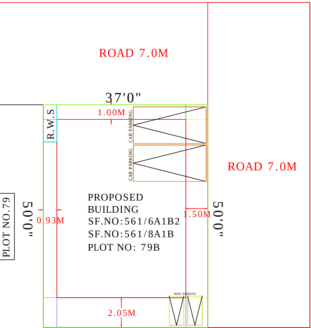
M.RAVINDRAN LAND SITE PLAN SCALE 1:100
