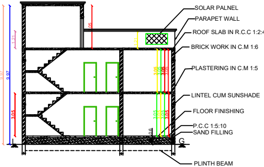
SECTION A-B
