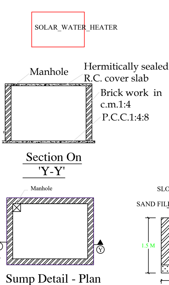
SUMP_CAPACITY_L=1000LTRS
