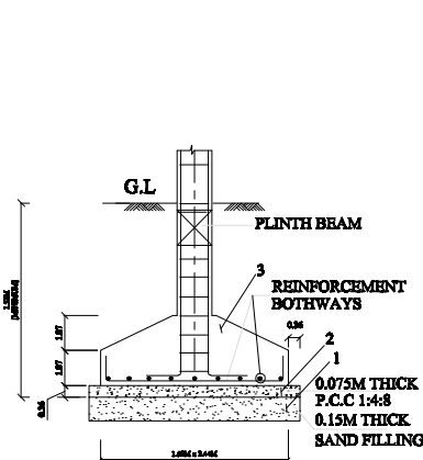
TYP. DET. COLUMN FOOTING
