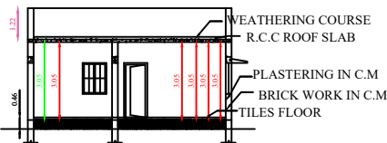
SECTION 'ab'
