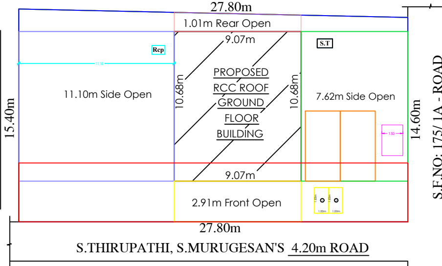
SITE PLAN 1:100
