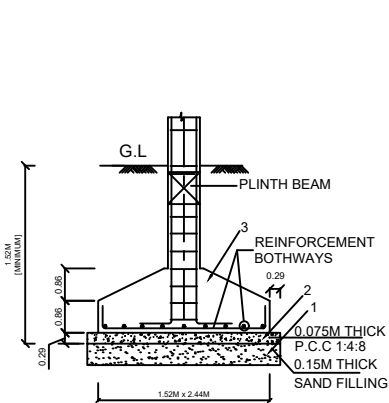
TYP. DET. COLUMN FOOTING
