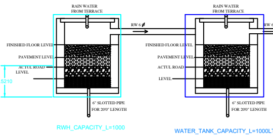
RW_CAPACITY_L=1000 WATER_TANK_CAPACITY_L=1000LTRS
