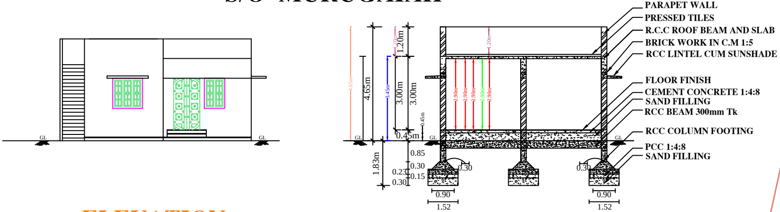
ELEVATION
