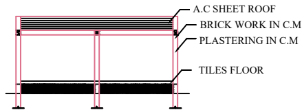
SECTION 'ab'
