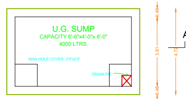
SUMP DETAIL SCALE: 1\"/>
