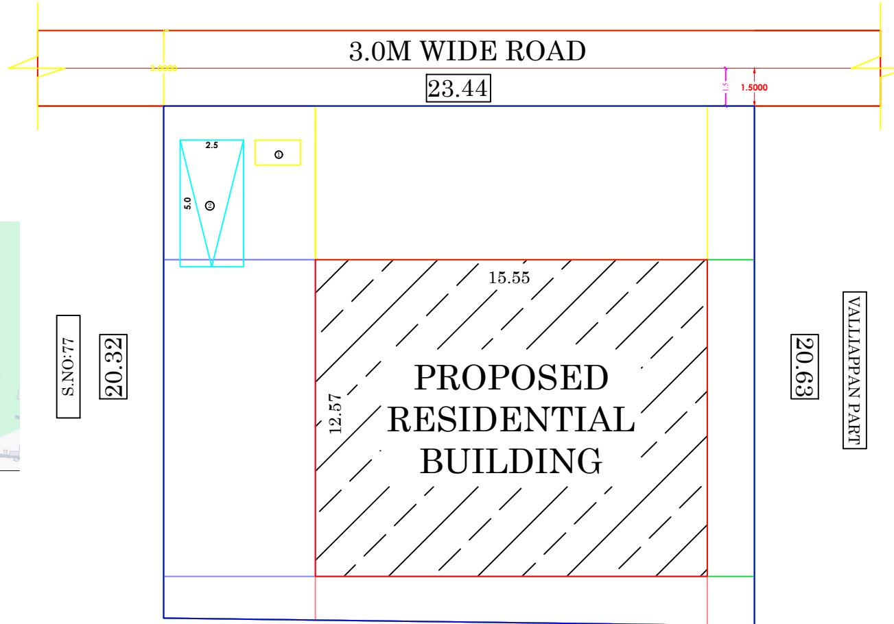
KEY PLAN - 10°15'07.3"N 78°39'27.8"E
