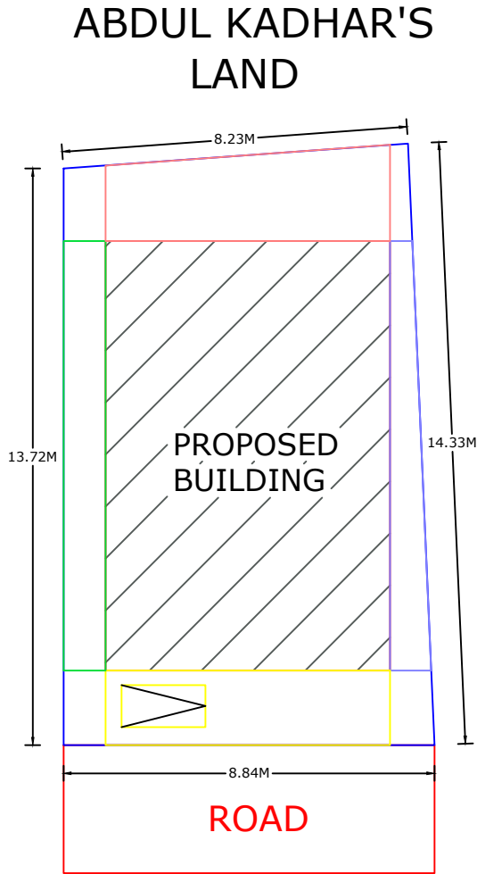
SITE PLAN: 1:100
