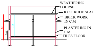
SECTION 'ab'
