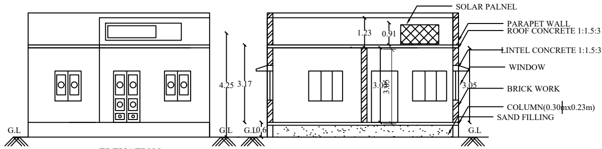
ELEVATION
