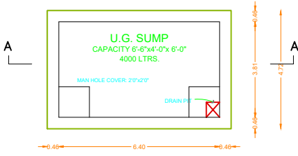
U.G. SUMP
