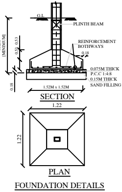
TYP. DET. COLUMN FOOTING
