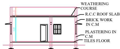
SECTION 'ab'
