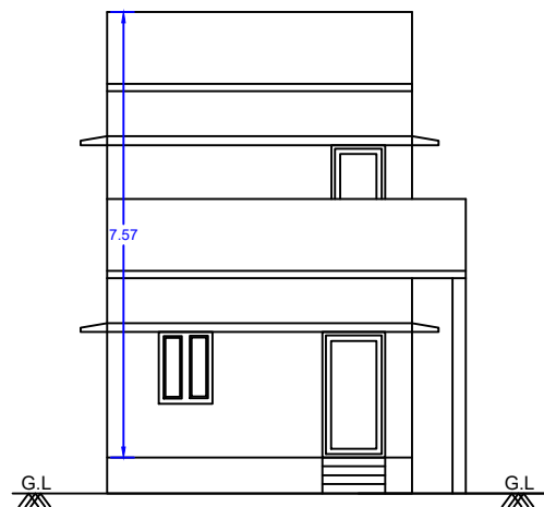
ELEVATION
