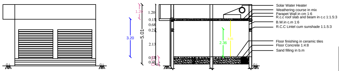
ELEVATION
