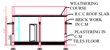
SECTION 'ab'
