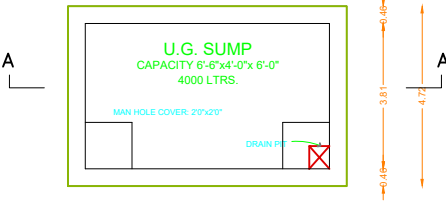
SUMP DETAIL SCALE: 1"=2'-0"
