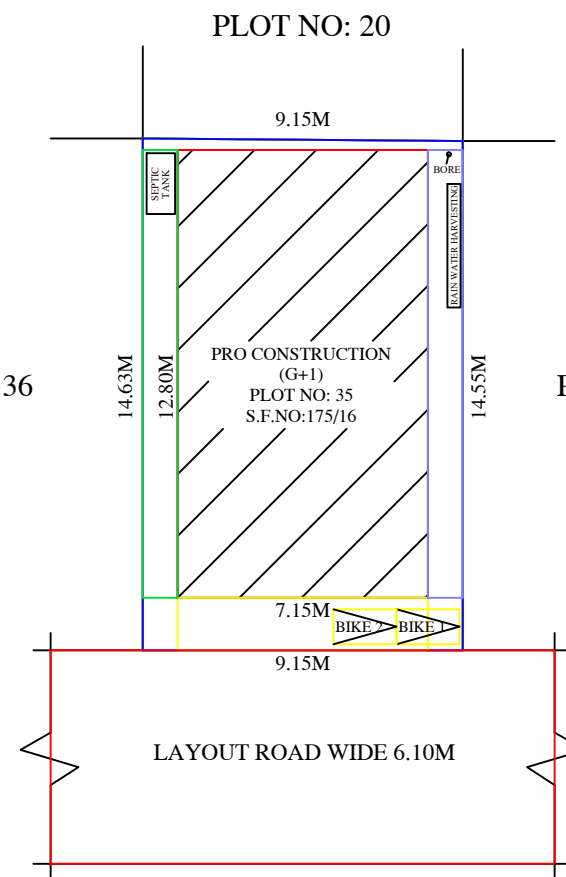
SITE PLAN:-
