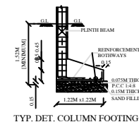
TYP. DET. COLUMN FOOTING
