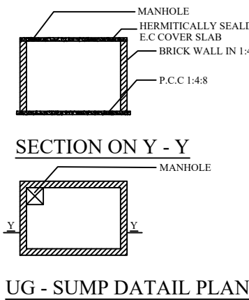
UG - SUMP DATAIL PLAN
