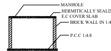
SECTION ON Y - Y
