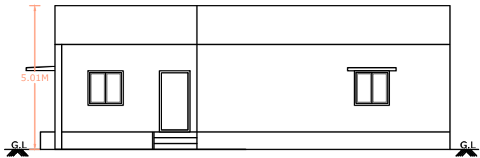
ELEVATION
