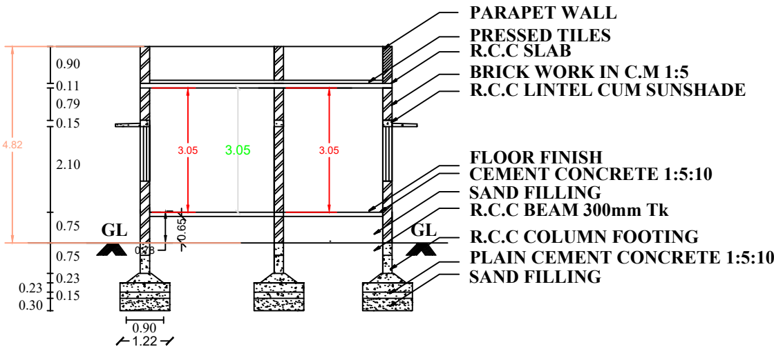
SECTION (A-A)
