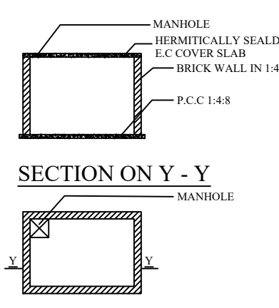
UG - SUMP DATAIL PLAN
