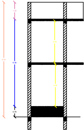
SECTION A-B
