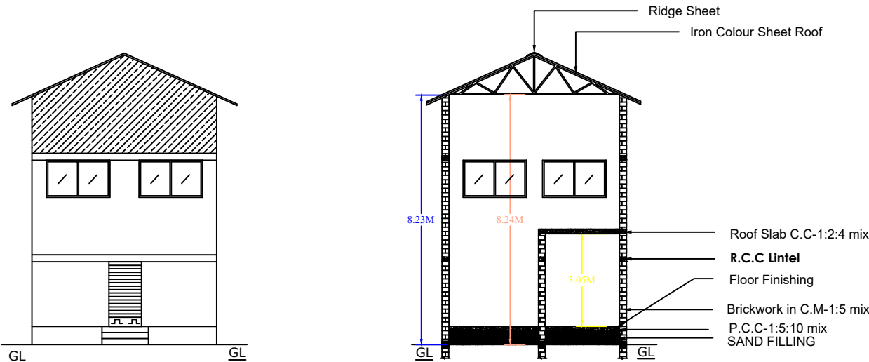
ELEVATION
