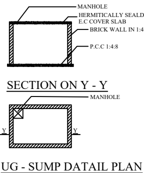
UG - SUMP DATAIL PLAN
