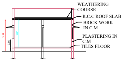
SECTION 'ab'
