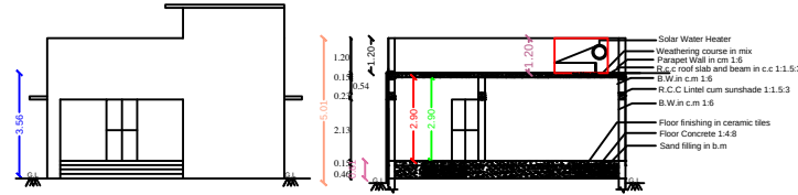
ELEVATION
