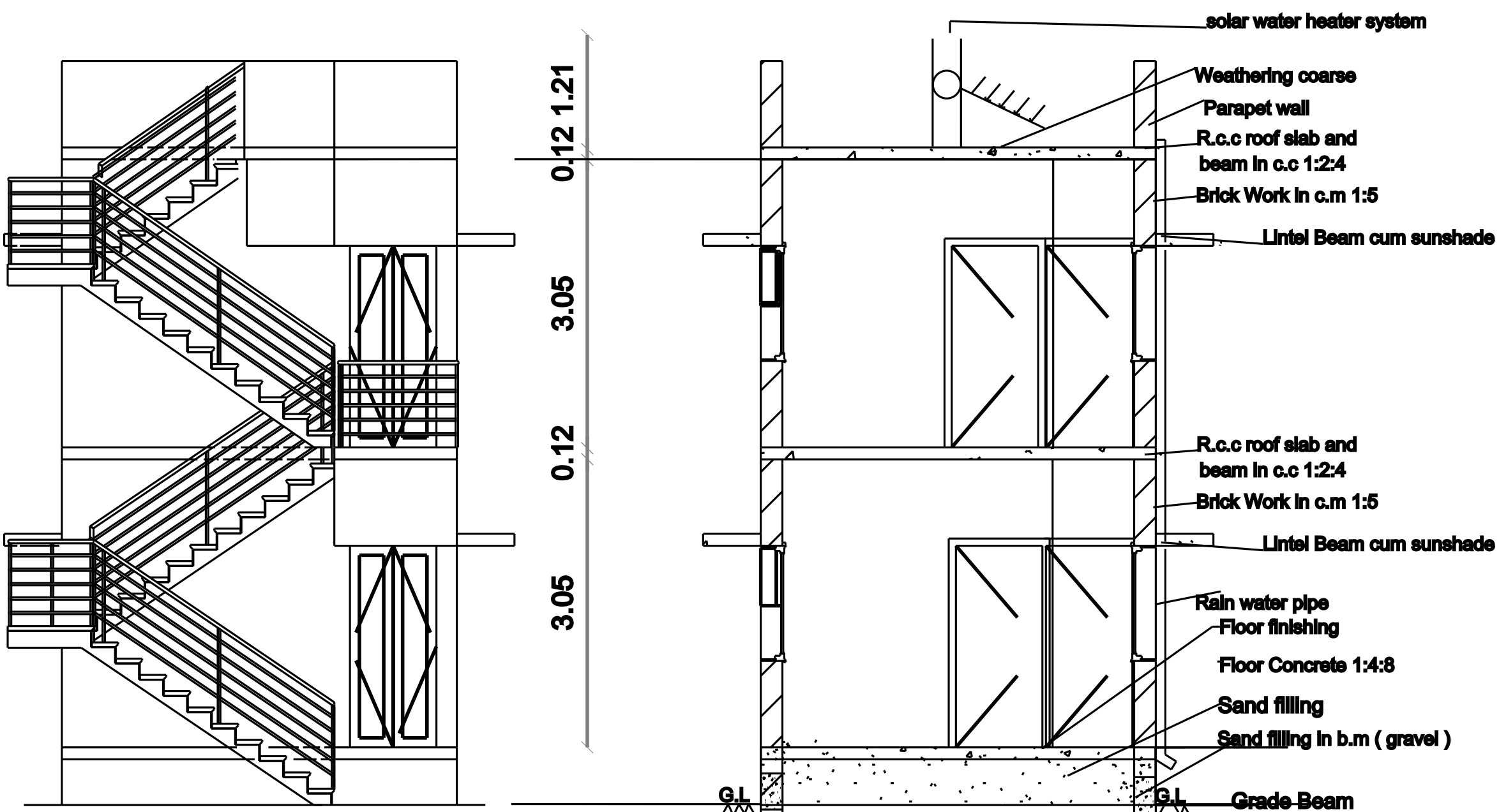
ELEVATION
