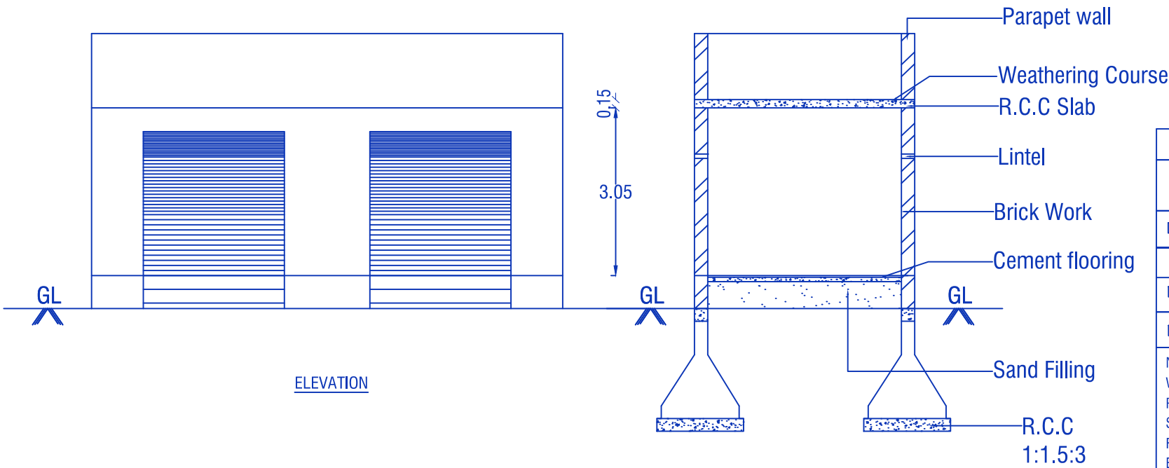
SECTION ON'AB'
