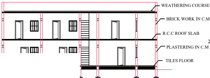
ELEVATION
