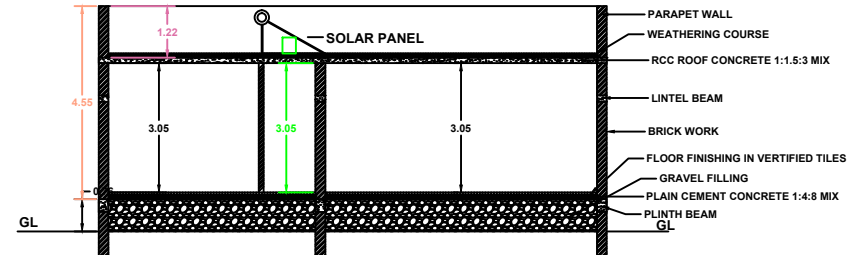
SECTION 'AB'
