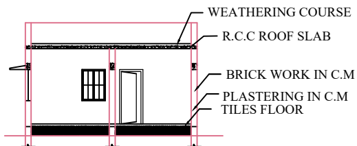
SECTION 'ab'
