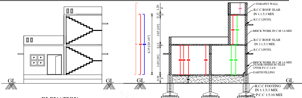
ELEVATION
