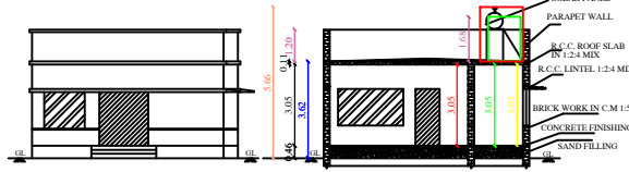
ELEVATION
