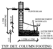
TYP. DET. COLUMN FOOTING
