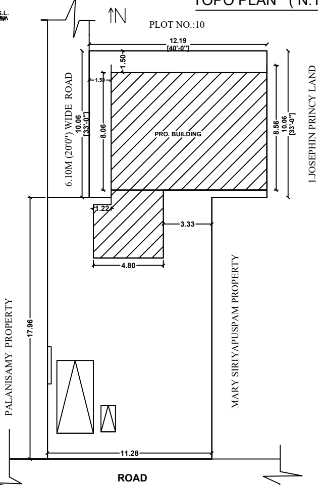
TOPO PLAN ( N.T.S)
