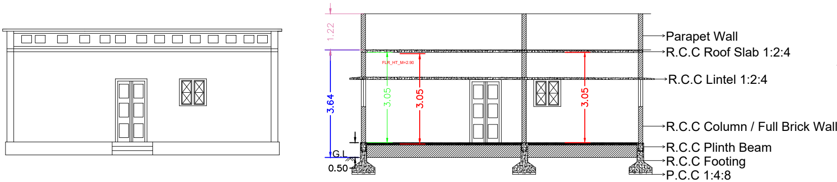
ELEVATION
